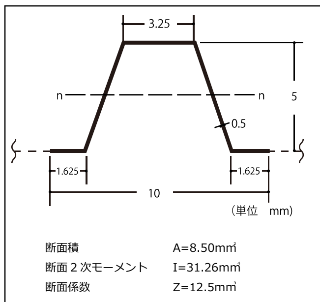
スーパードフォーム使用例 板厚0.5
